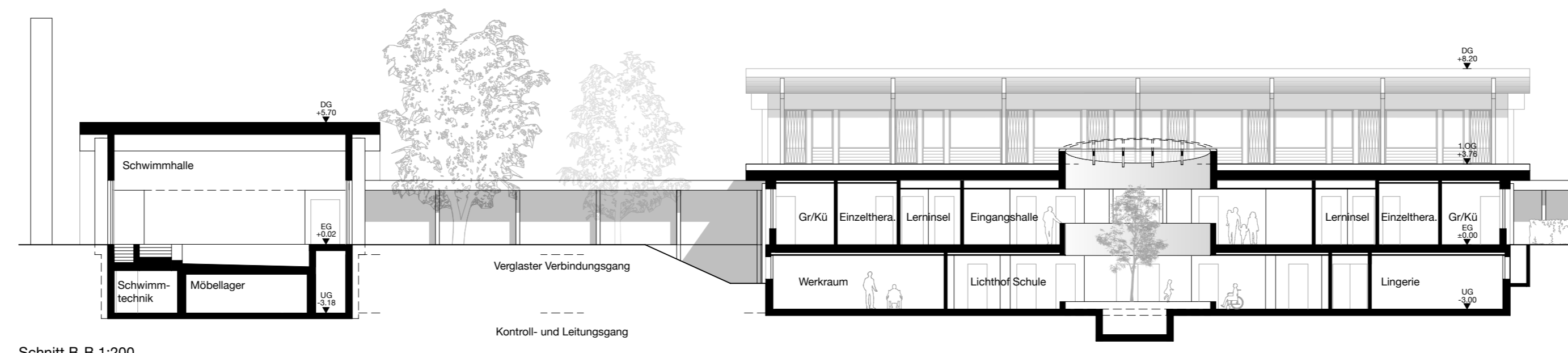
Schnitt B-B 1:200
